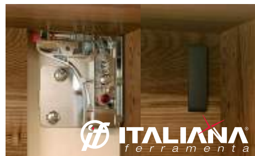
Detalle Colgador y Tapa decorativa interior
