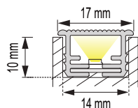
Montaje en canto exterior de Listón Trasero
