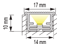
Montaje en canto exterior de Trasera
