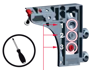
Detalle Regulaciones Colgador
