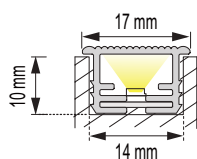
Montaje en canto exterior de Paneles
