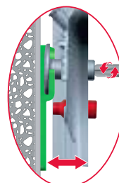
2. Ajuste Profundidad: 12 mm
