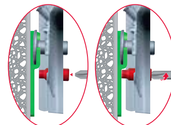
3. Detalle Sistema Antidescolgamiento
